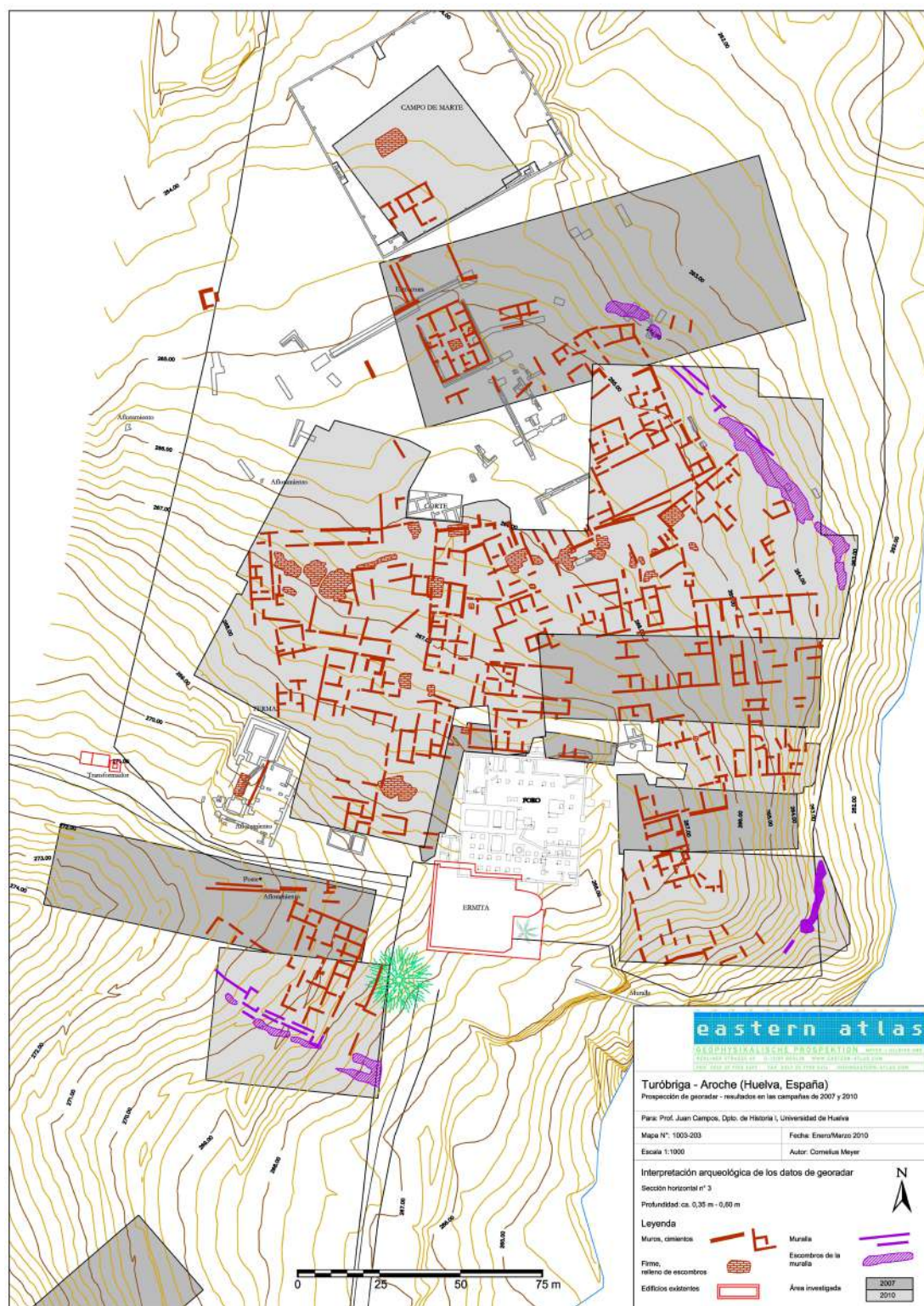
Fig. 46. Prospección geofísica mediante georadar (Universidad de Huelva).
