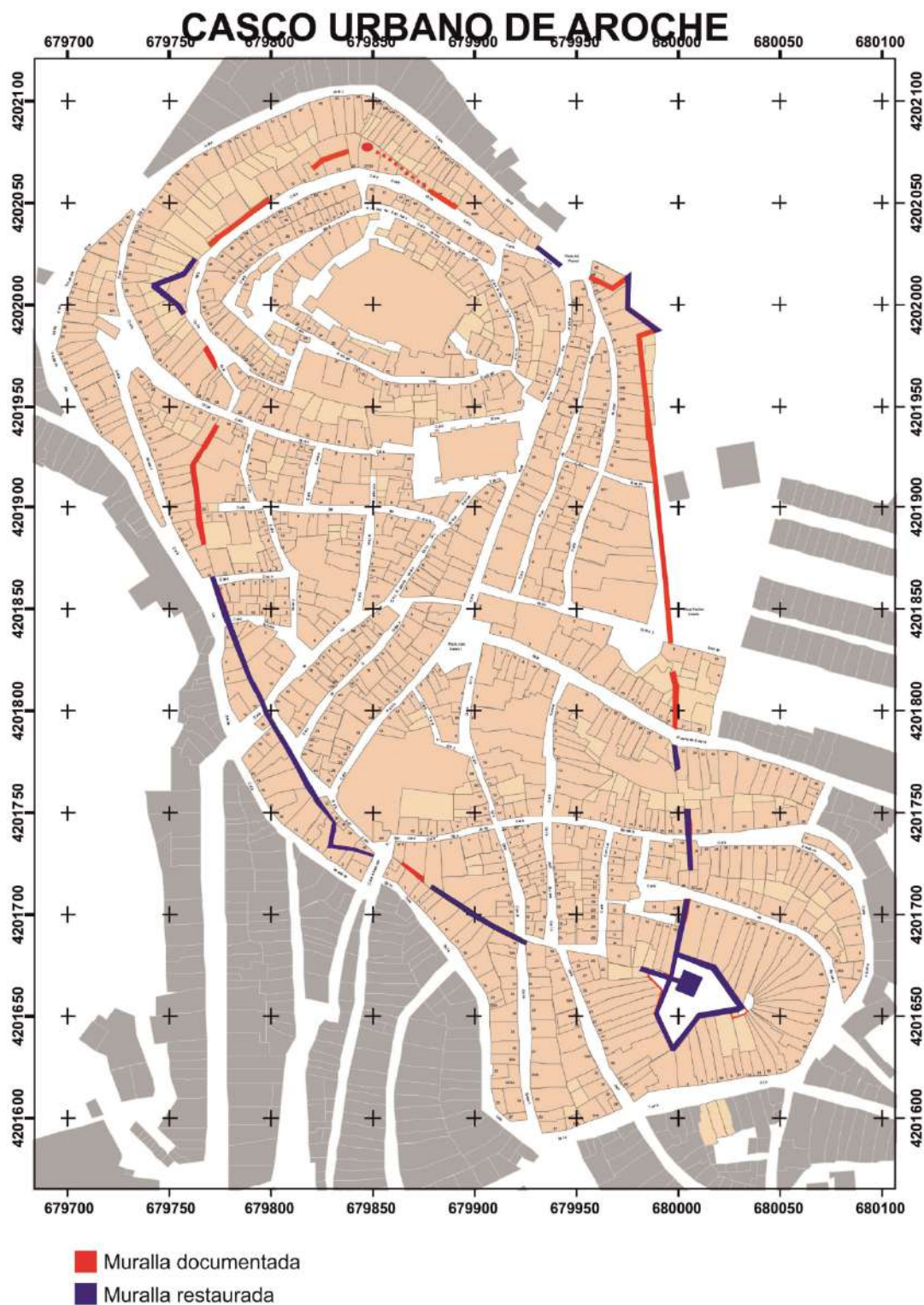
Fig. 87. Plano con indicación de los tramos de muralla documentados y restaurados (Ayuntamiento de Aroche).
