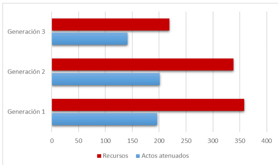
FIGURA 4. ATENUACIÓN SEGÚN EDAD. ADAPTADO DE SAMPER HERNÁNDEZ (2017)
