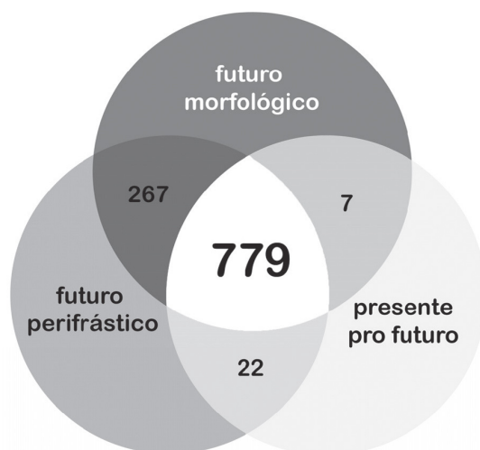
FIGURA 2. FRECUENCIA DE OCURRENCIAS Y CAPACIDAD DE NEUTRALIZACIÓN
