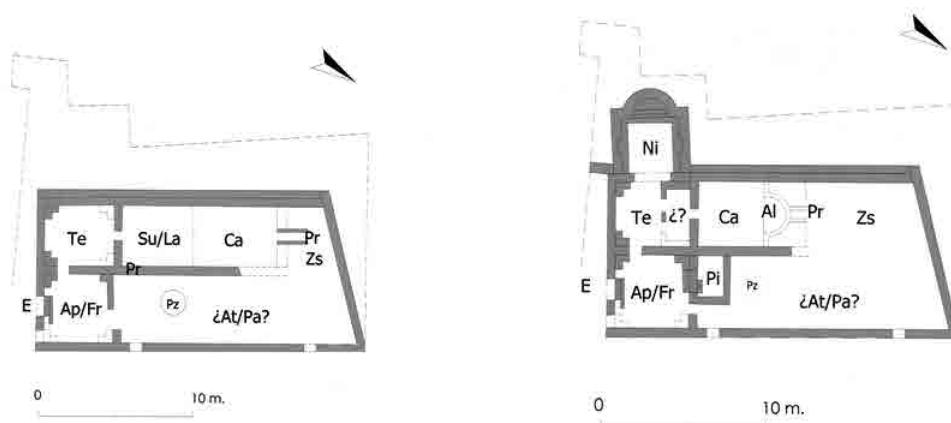
Figura 9. Vista general de las termas de Munigua con indicación de sus fases termales Iª, a Izquierda, y IIª, a derecha (según Gómez Araujo, 2013).
