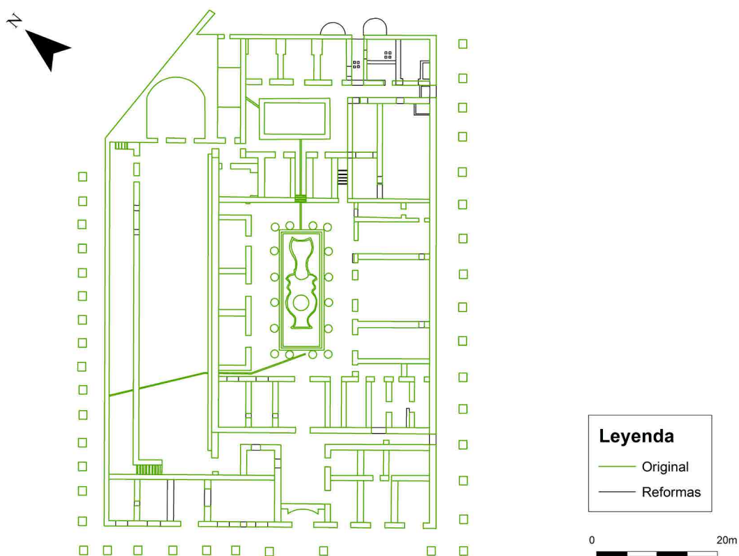
Figura 5: Planta de la Casa de la Exedra de Italica con indicación de la obra original y reformas (Elaboración propia, a partir de García-Entero e Hidalgo, 2016, fig.2 y Roldán Gómez, 1991, fig.11).
