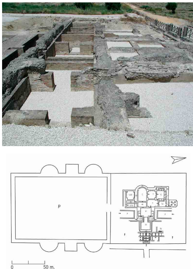
Figura 8. Vista general de las Termas Mayores de Italica con propuesta de articulación (según Gómez Araujo, 2008).
