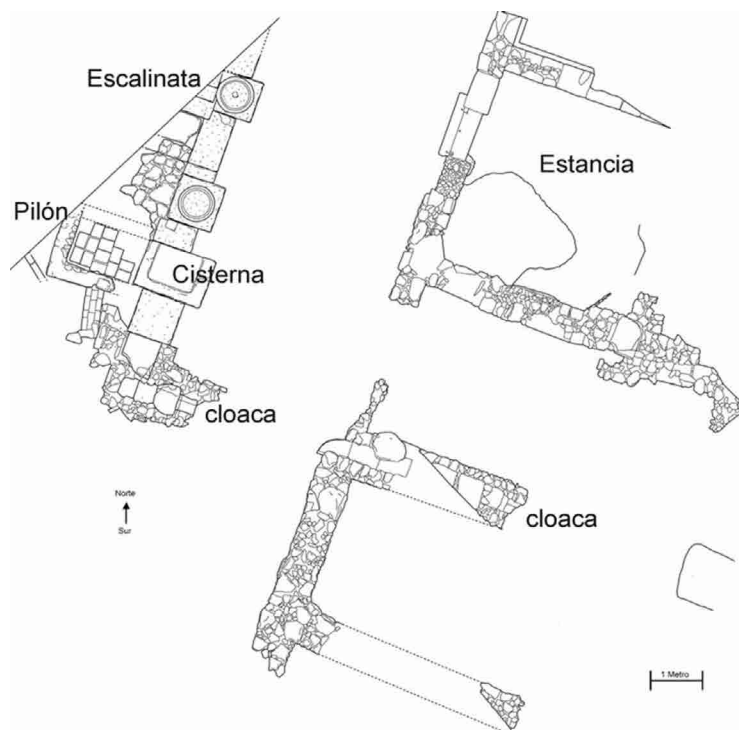
Figura 3. Planta del espacio porticado y las estructuras cercanas (Lineros y Márquez, 2014: 83, Figura 2)
