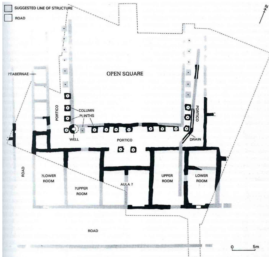
Figura 4. Plano interpretativo de las estructuras vinculadas con el foro (Keay et alii , 2000: 177, Fig. 9.1)
